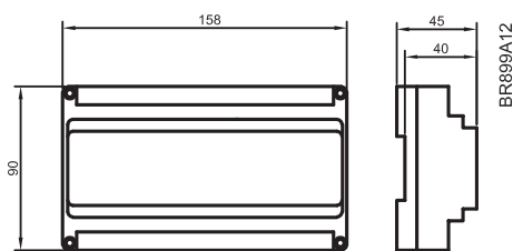
Размеры (мм)
